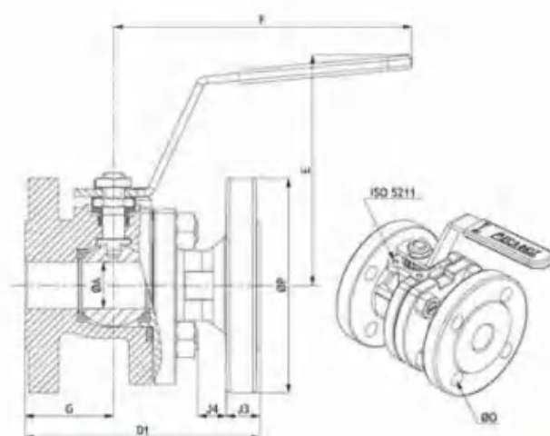
短结构 PN 40
