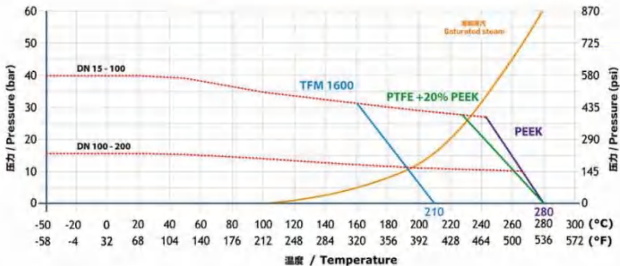
压力 / 温度图
